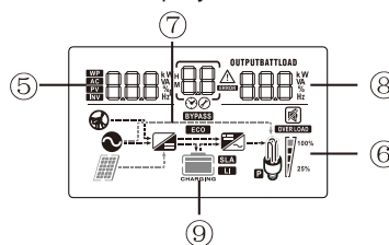
LCD display
